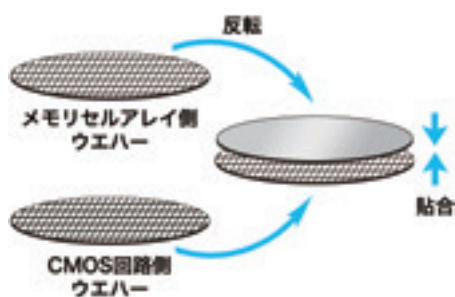
ウエハーを貼り合わせる CBA(CMOS directly Bonded to Array)技術
