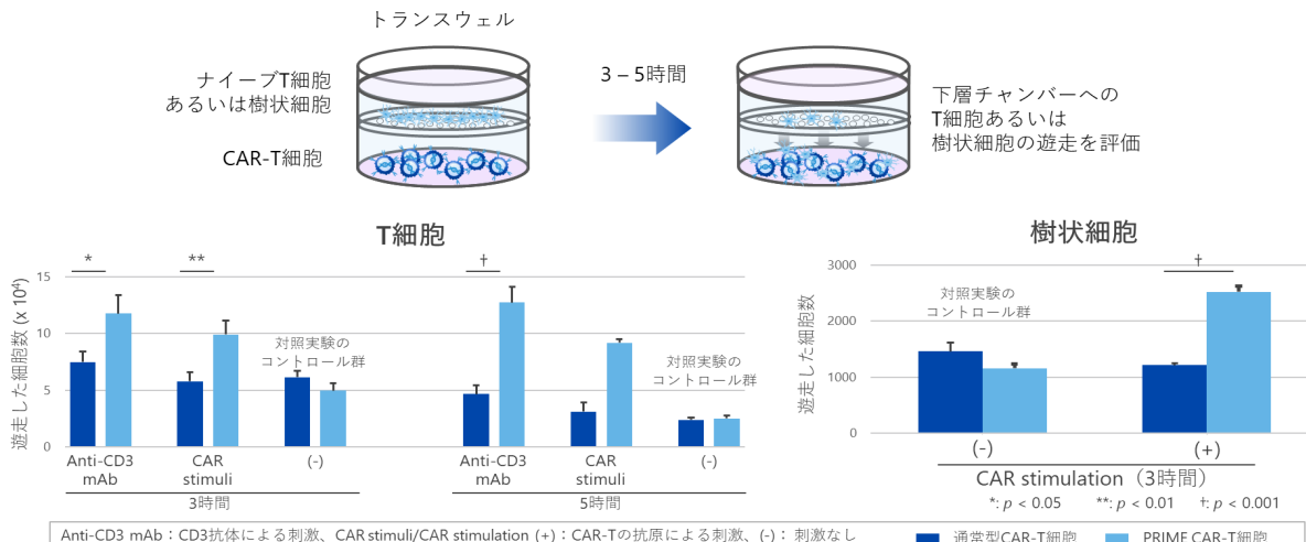
図5. CCL19の効果を確かめる細胞遊走試験
